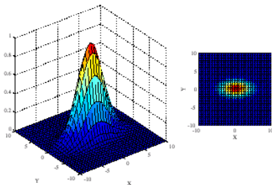
Funkcja Gaussa wielu zmiennych
